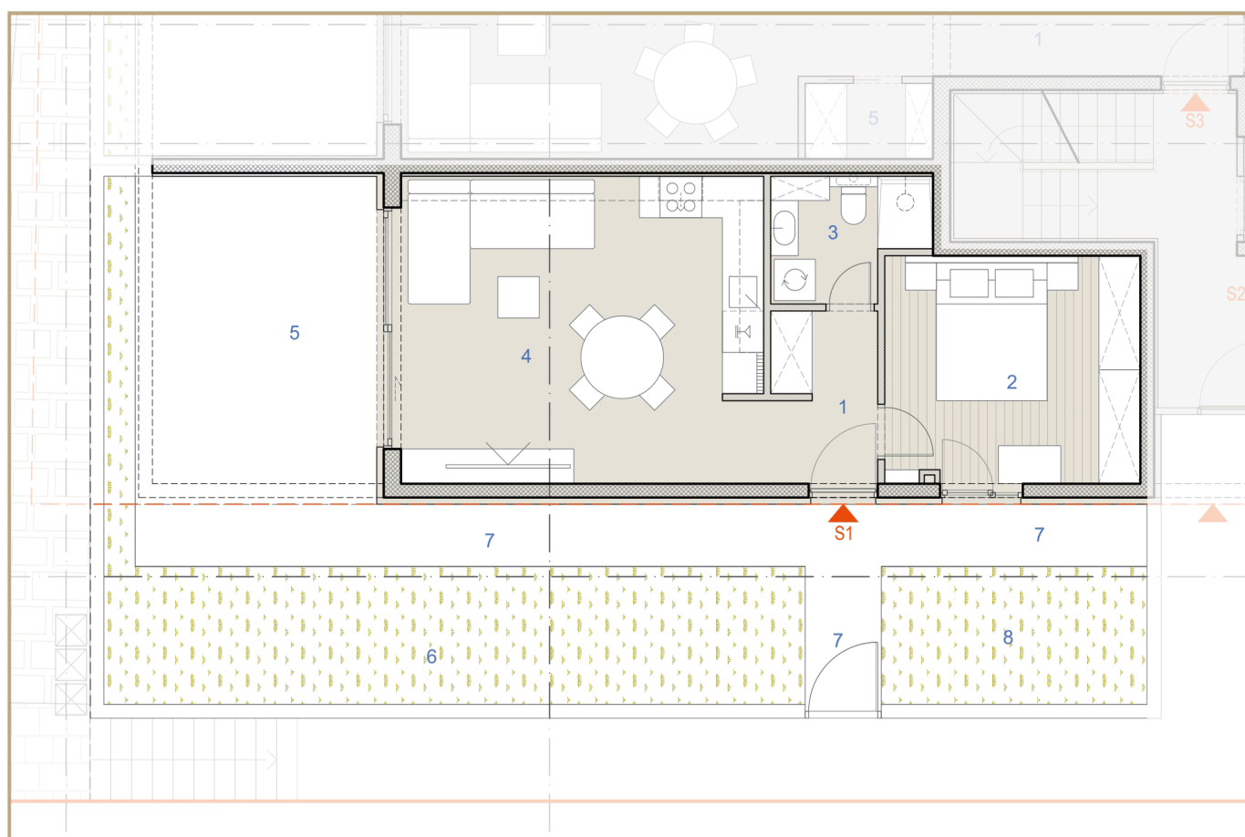
Zgrada Zapad - prizemlje - stan S1
